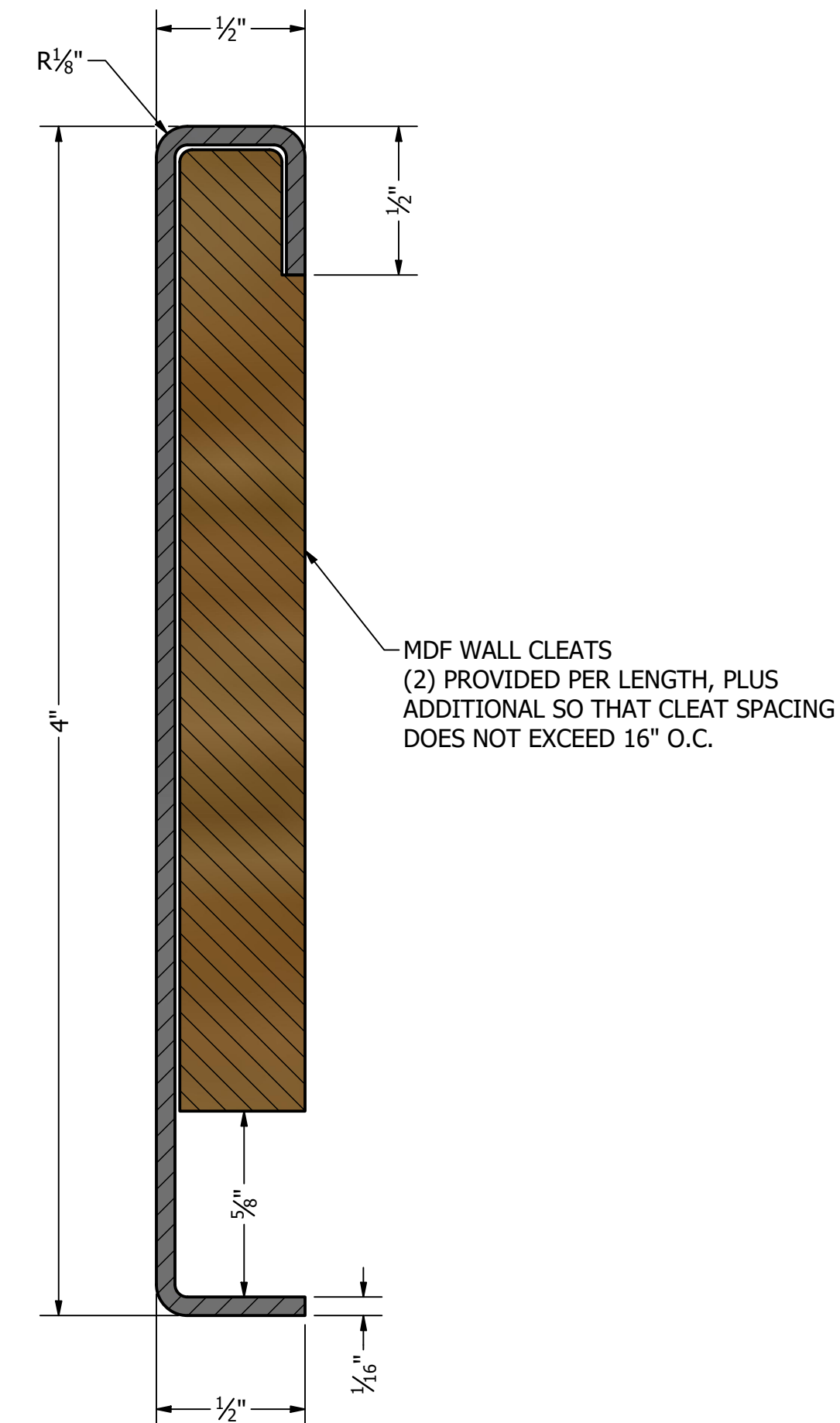
SECTION A-A SCALE 2 : 1
